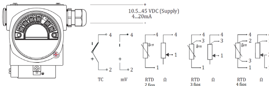
Figura 2 – Ligação elétrica MST885
