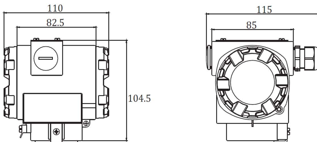
Figura 13 – Desenhos dimensionais MST885
