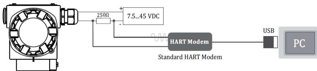
Figura 12 – Operação com modem HART
